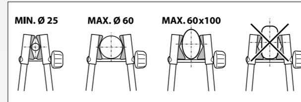
GOMMINO SALVATELAIO RUBBER TUBE PROTECTOR
