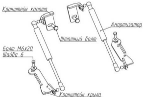
Схема установки
